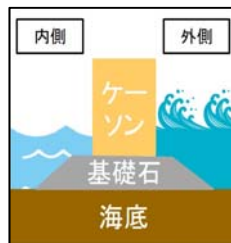
防波堤断面図 (イメージ)
