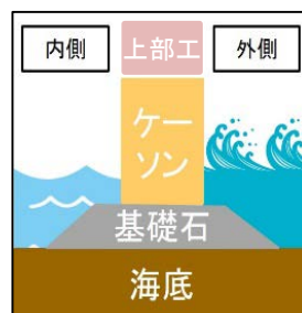
防波堤断面図 (イメージ)
