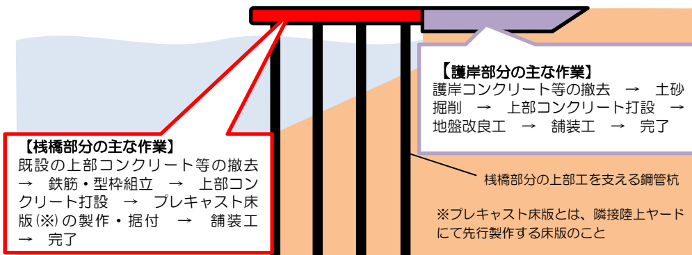
地盤改良のための土砂掘削
