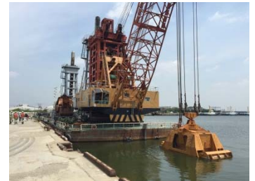
▲今回見学した浚渫船
