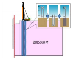
施工断面
